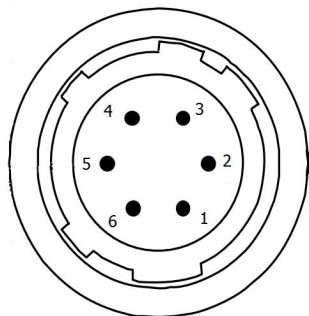
图 2 外触发接口
