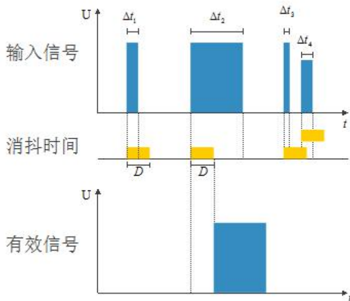
图 6 信号消抖
