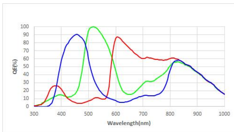
图 1 光谱响应图
